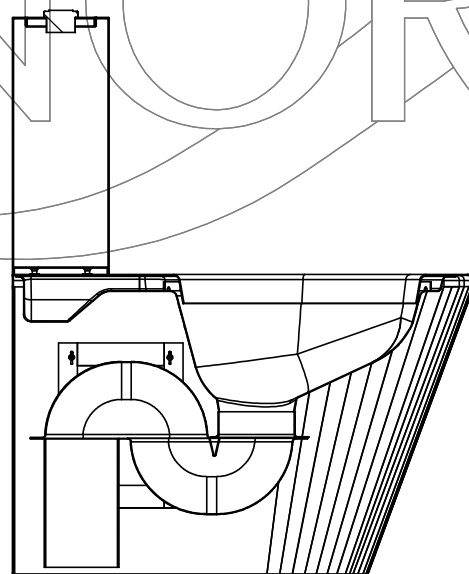
KESIT A-A
